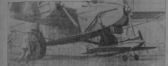
En esta fotografía vemos al monoplano más pequeño del mundo al lado de un gigantesco avión. Ambos aparatos son pertenecientes a la Fuerza Real Aérea de Inglaterra, tomándose esta foto durante una maniobra efectuadas recientemente en Hendon, Inglaterra.
